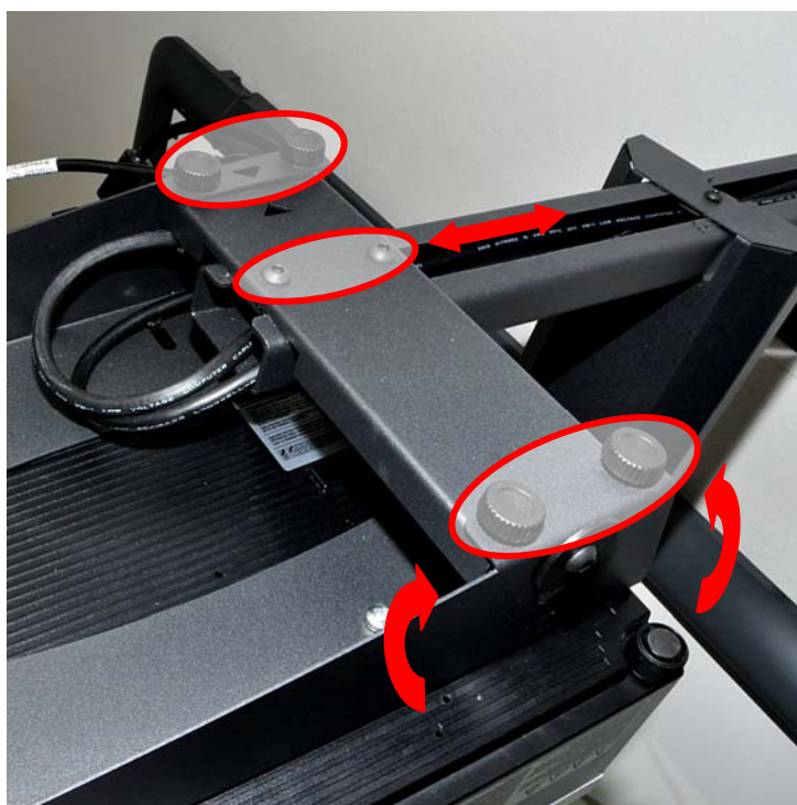
Nastavenie polohy projektora (veľkosť a pozícia obrazu na tabuli)
