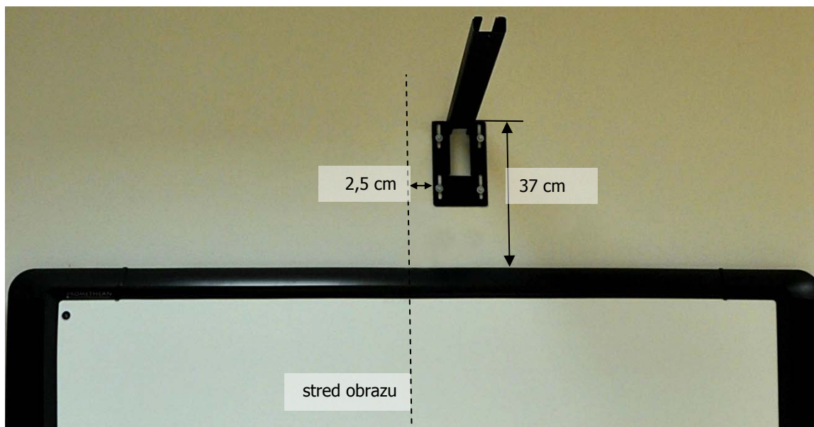
Poloha základne nástenného ramena voči interaktívnej tabuli
